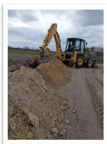
Wymiana hydrantów zewnętrznych, budowa sieci wodociągowej, budowa zbiornika wody czystej (fot. UG Włocławek)
